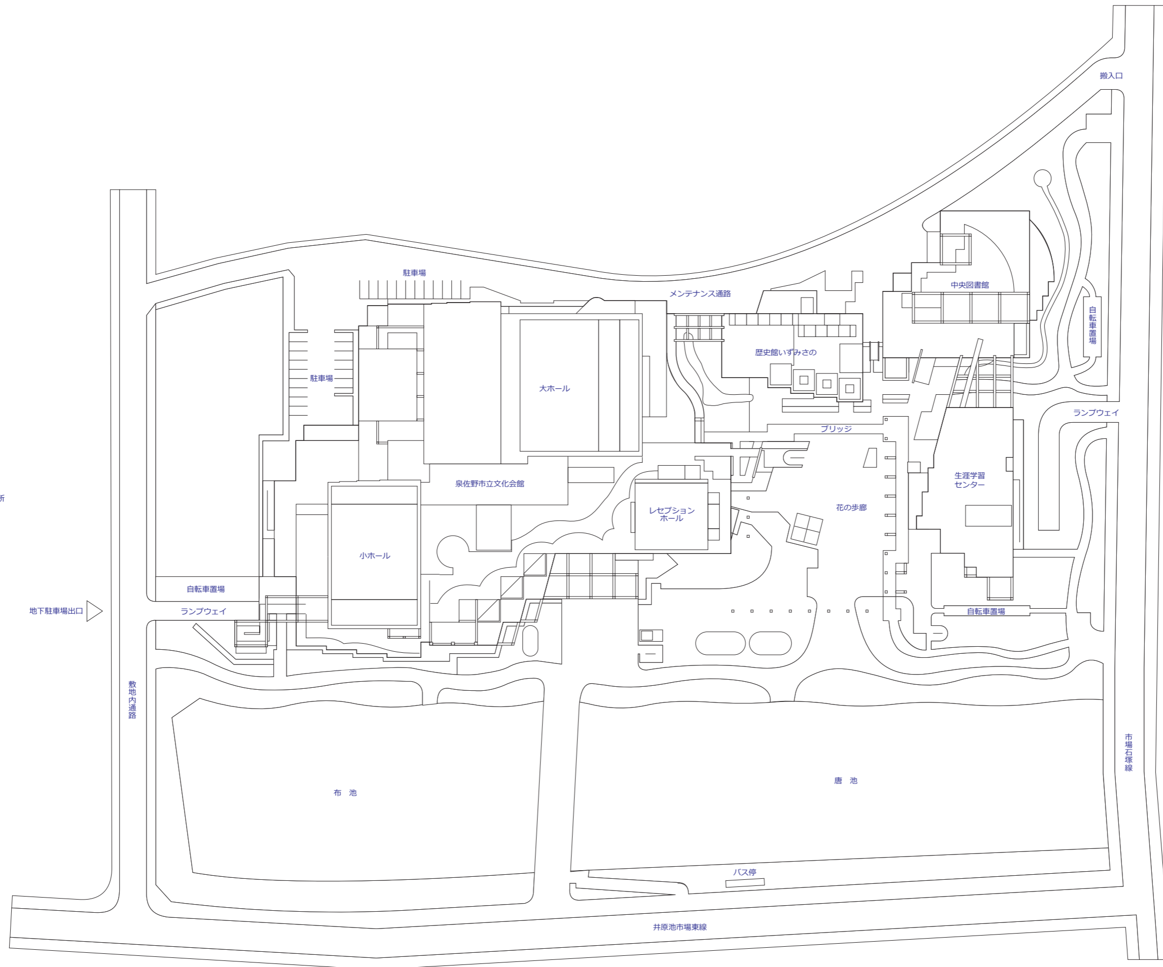
泉佐野市立文化会館 配置図 S:1/1000 0 10 20 30 50(m)
